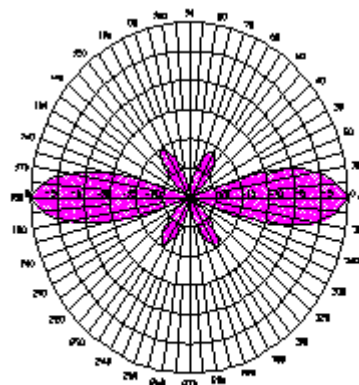
垂直方向图
